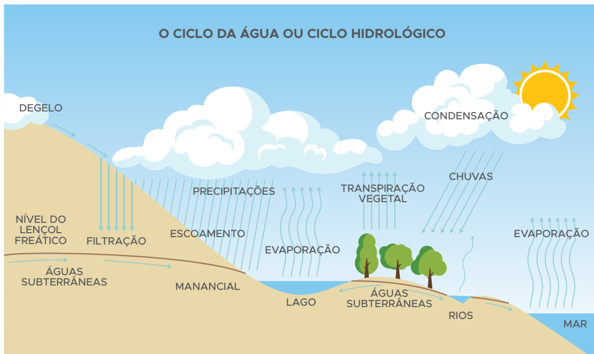
Ciclo global da água ou ciclo do hidrológico. Fonte: Elaborado para fins didáticos.
